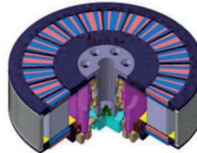
[PAV용 고출력 모터]
